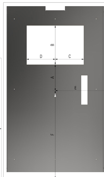
Monitor Außenmaße External dimensions
