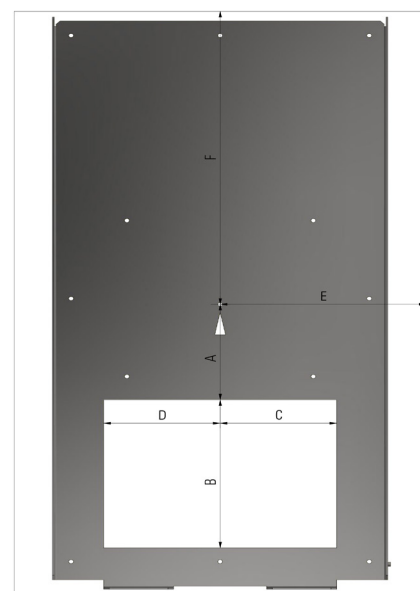
Monitor Außenmaß External dimensions
