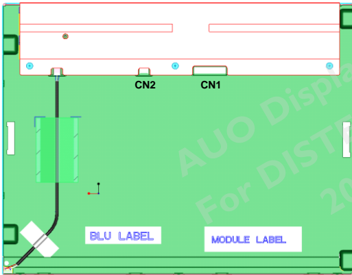
LVDS(CN1):
